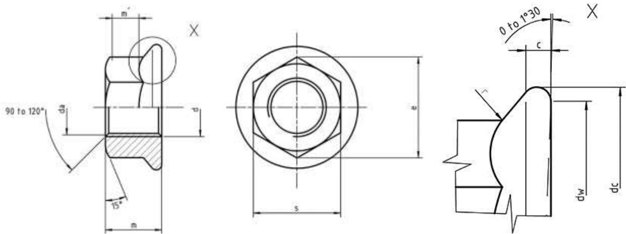
Dimensions of Metric DIN 6923 Hexagon Flange Nuts
