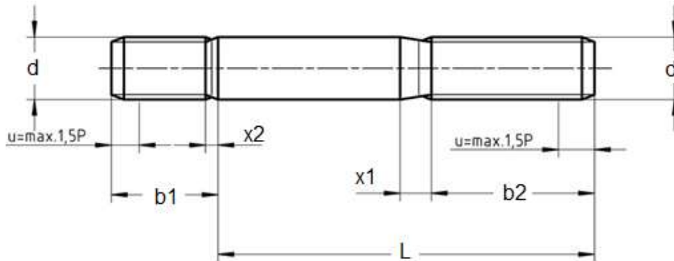
Dimensions of Metric DIN 938 Double End Studs
